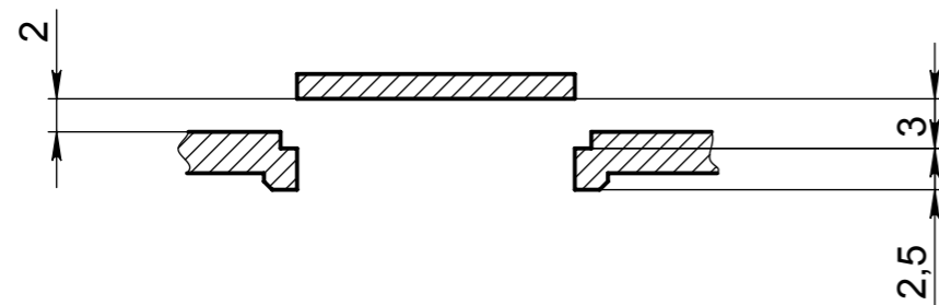
A-A (2 : 1)
