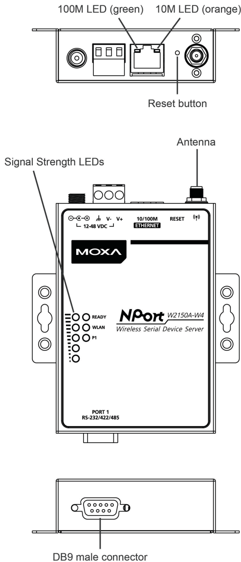
NPort W2150A-W4/W2150A-W4-T
